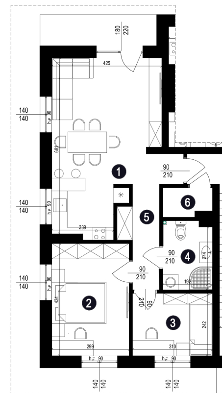
Rzut mieszkania
