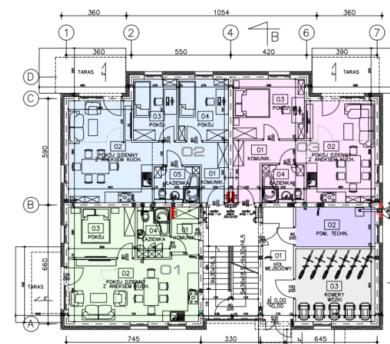
LOKAL 03 PARTER
