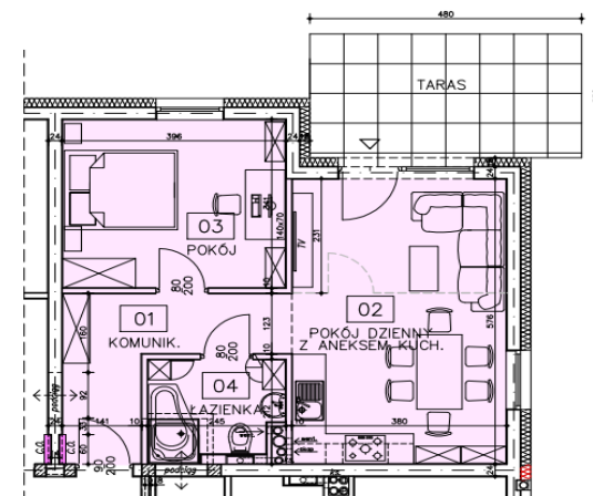
LOKAL 03 PARTER
